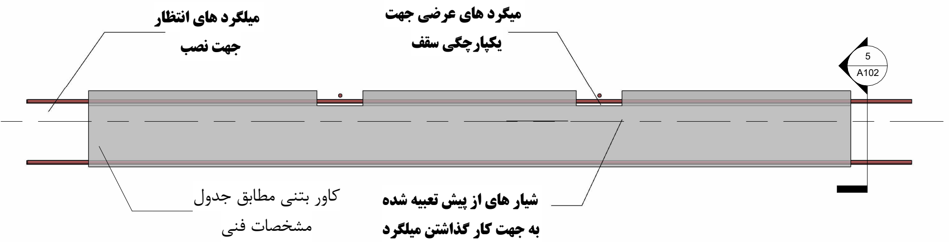
2 نمای طولی سقف 1 : 11
