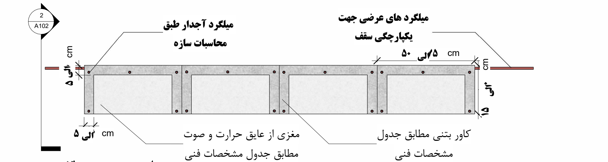
5 نمای عرضی سقف 1 : 11
